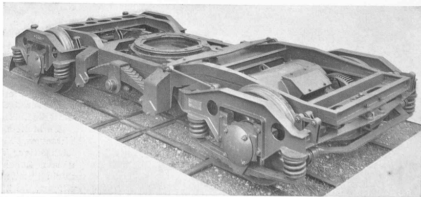
Abb. 2. Liechty-Lenkdrahgestell mit 3400 mm Radstand, erbaut von der S. I. G. Neuhausen
