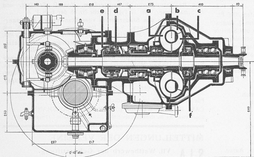
Abb. 2. Trilokgetriebe für Dieseltriebwagen. — a Pumpenrad der Antriebsseite, b Turbinenrad der Abtriebsseite, c Leitapparat, d, e Gesperre, f Freilauf zwischen Turbinenrad und Abtriebswelle.
