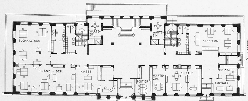
Abb. 4. Erdgeschoss-Grundriss.
