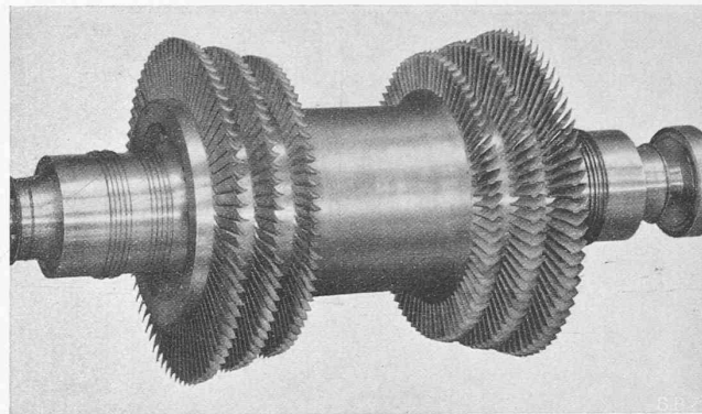
Abb. 8. Rotor einer Gasturbine mit Reaktionsbeschaufelung.
