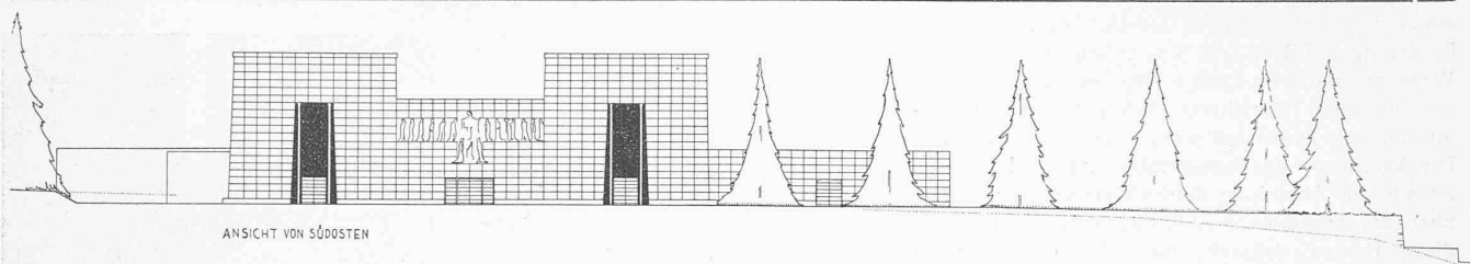
Ankauf (3000 Fr.), Entwurf Nr. 34. — Verfasser Gebr. Bräm, Architekten, Zürich. — Südost-Ansicht 1 : 600.
