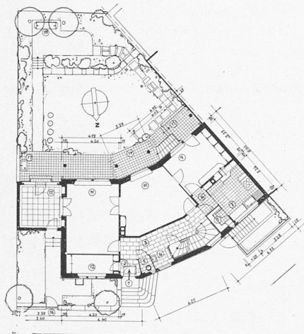
Abb. 21. Erdgeschoss.
