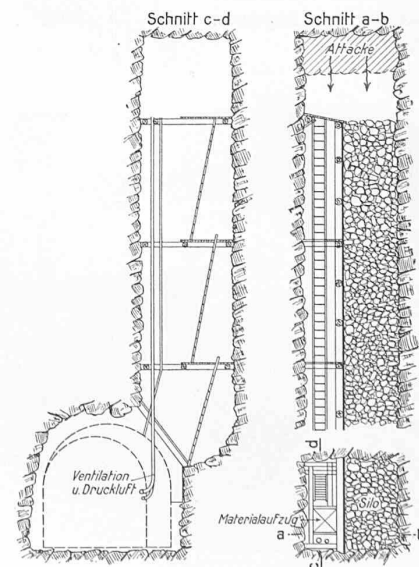
Abb. 12. Ausbruchvorgang der Schächte. — 1 : 200.
