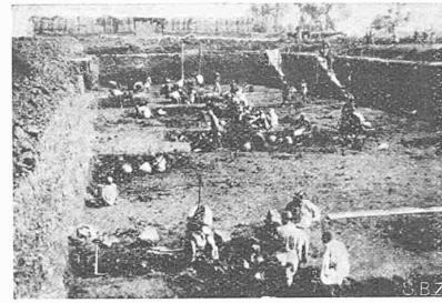
Abb. 4. Aushub und Transport von Hand für die Fundamente des Kraftwerkes Minieh (Ägypten).
