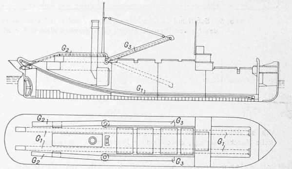
Abb. 7. Kohlentransportdampfer „Pallion“ mit Gurtförderanlage. — 1:1000.
