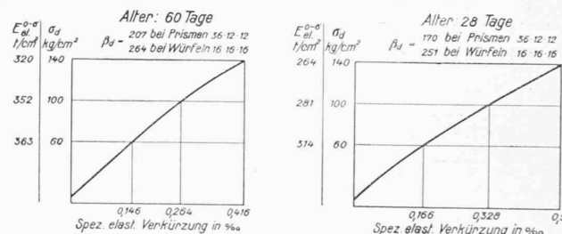
Abb. 14. Elastizitätsmessungen an Betonprismen 12x12x36 cm. Normal P.-Z.-Marke 8. — 250 kg Z. auf 1 m 3 Kies-Sand (1:2). Wasserzusatz 6,5% des Trockensubstanz-Gewichtes.
