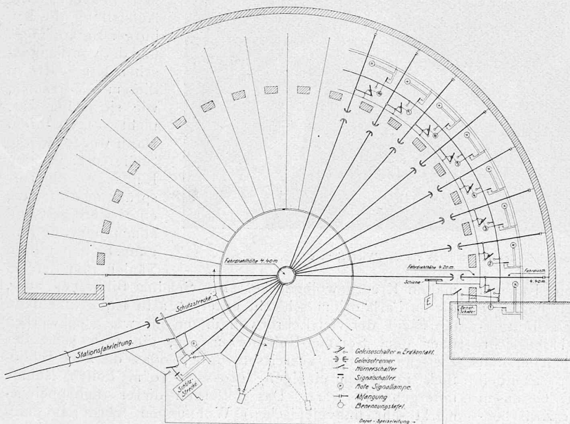
Abb. 9. Schaltungschema der Fahrleitungsanlage des Lokomotivdepot Landquart.
