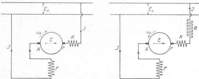
Abb. 7. Einphasen-Seriemotor mit Armatur A, Feld F, Kompensationswicklung K und Seriawicklung r, als Motor (links) und als Gegenstrombremse (rechts) mit Bremswiderstand R.
