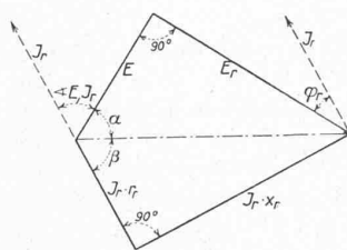
Abb. 10. Spannungsdiagramm des Einphasen-Seriemotors für die Schaltung nach System Oerlikon wie Abbildung 9, bei Wirkungsweise der Maschine als Motor.
