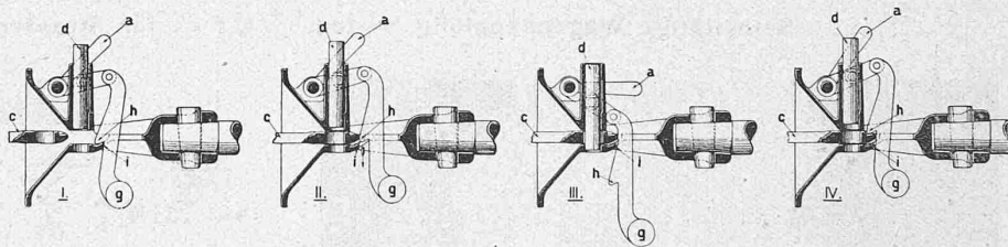
Abb. 4. Schematische Darstellung des Kupplung-Vorganges; IV. Entkuppeln.
