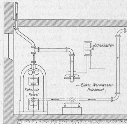
Abb. 3. Schema einer Warmwasser-Zentralheizungsanlage mit elektrisch geheiztem Hilfskessel von etwa 30 kW.
