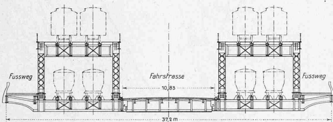
Abb. 13. Fahrplan der Manhattan-Brücke.
