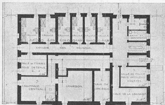
Plans des étages. — Echelle 1:400.
