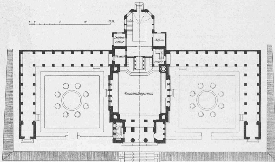
Grundriss des Krematoriums mit Urnenhallen. — Masstab 1:400.
