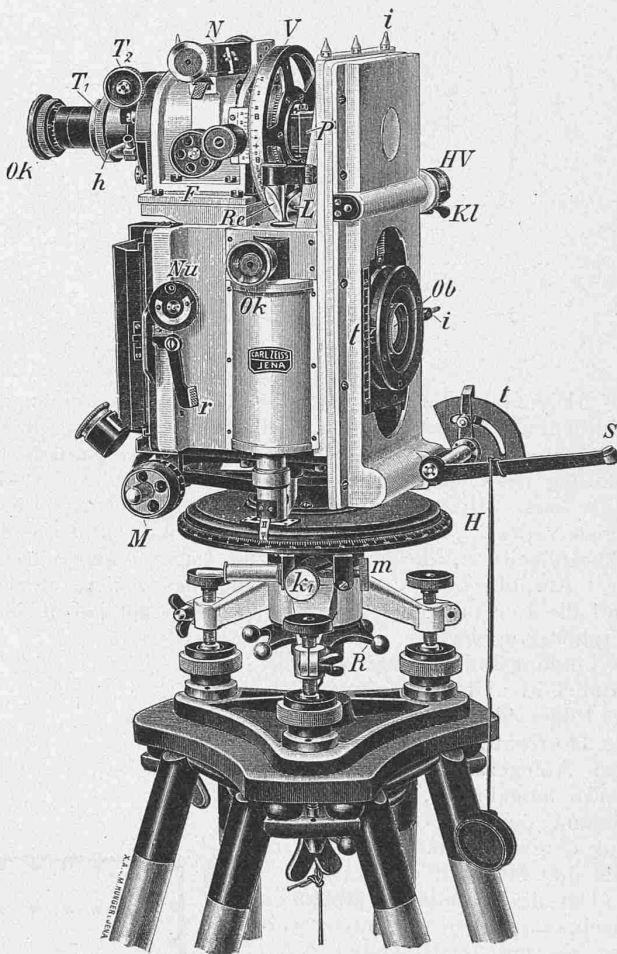
Abb. 7. Phototheodolit von Carl Zeiss, Jena; für Plattenformat 9 \times 12 ; Brennweite 127 mm.
