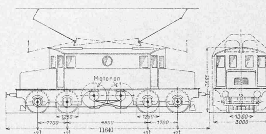
Abb. 5. Lokomotive der Simplonbahn, gebaut 1907
