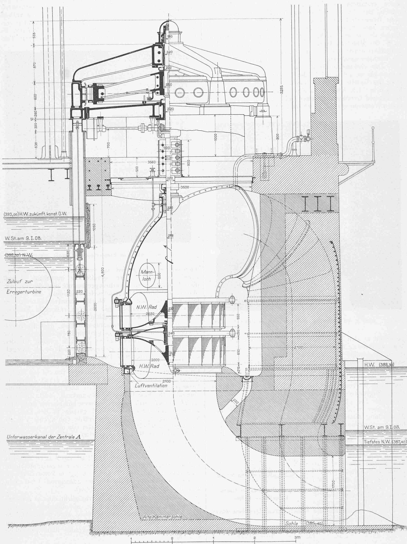
Abb. 10. Vertikalschnitt durch die 550 PS-Doppelfrancis turbine mit Generator in der Zentrale B. — Masstab 1:50.
