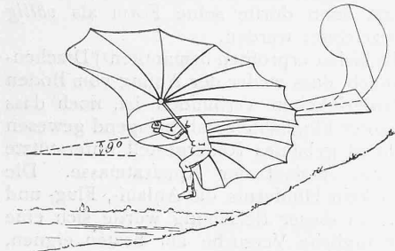
Abb. 10. Lilienthals Gleitflieger.
