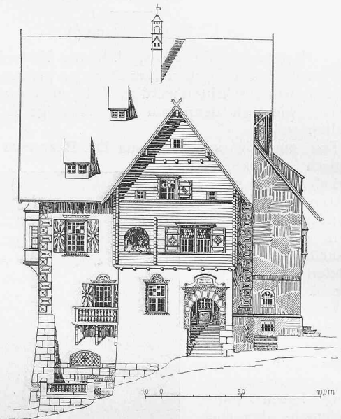
Abb. 5. Ostfassade mit Eingang für die Patienten.
