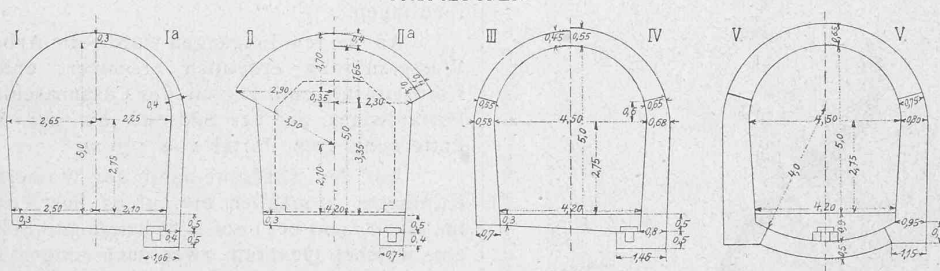
Abb. 10. Normalquerschnitt des Albulatunnels.
