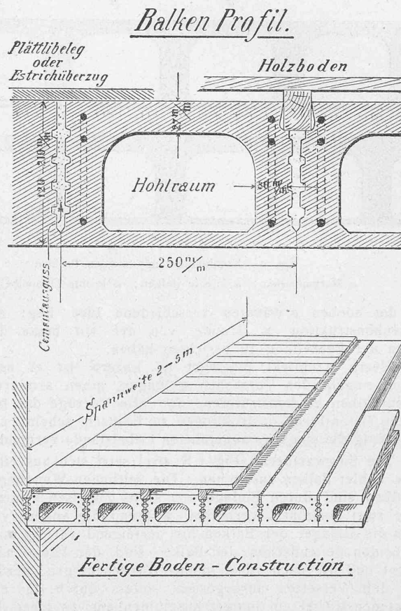
Fig. 1. Siegwartdecke.
