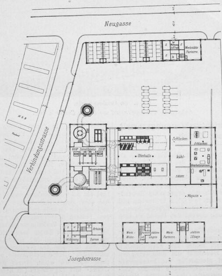
Fig. 1. Grundriss. 1:1000.
