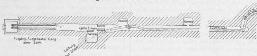
Fig. 19. Grundriss des Südstollens der Wasserleitung von Samos.
