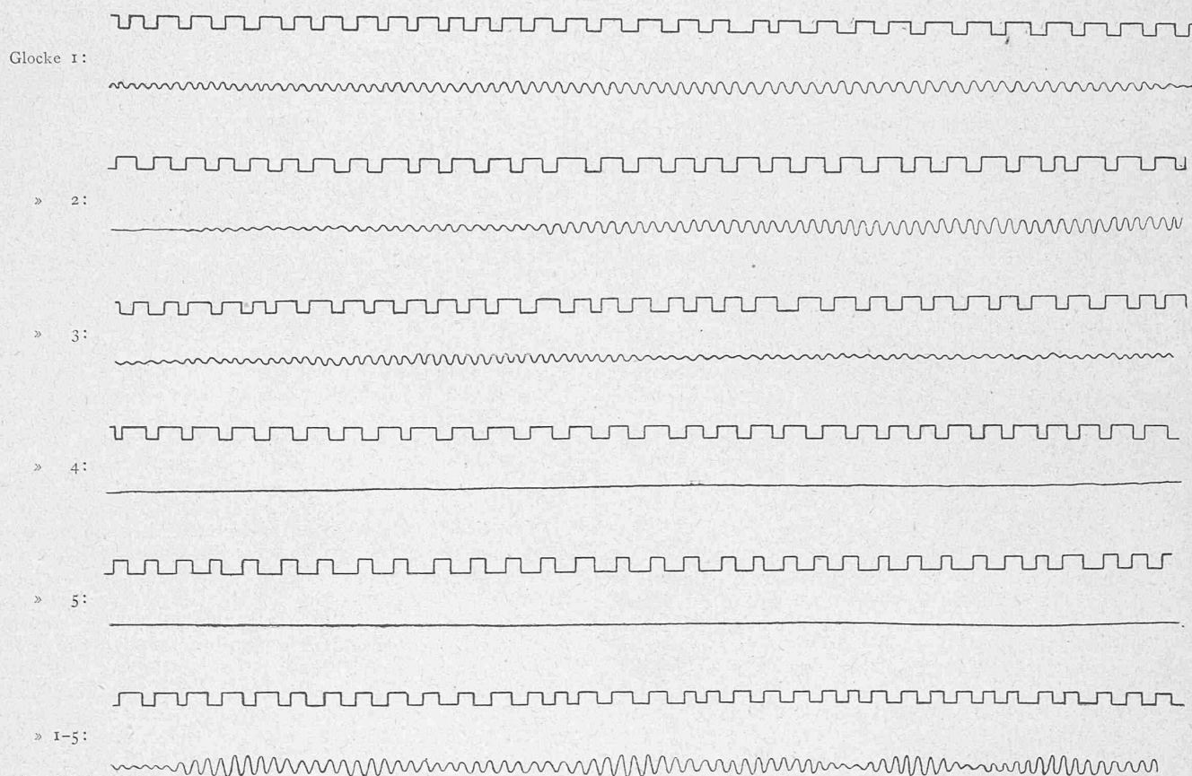
Fig. 2. Querschwingungen (Ost-West).
