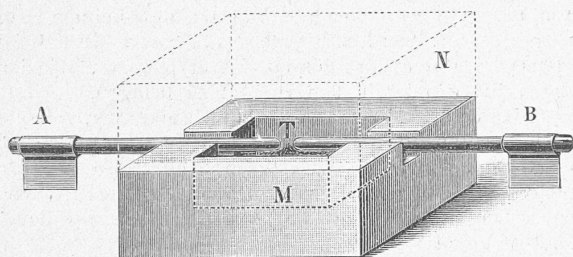
A und B Elektroden aus Kohle. M Steinblock aus weichem Kalkstein. N Steinplatte » » » T Vertiefung für den Kohlentiegel
