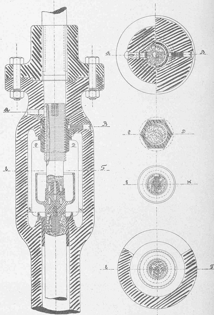
Spurzapfen und Welle.
