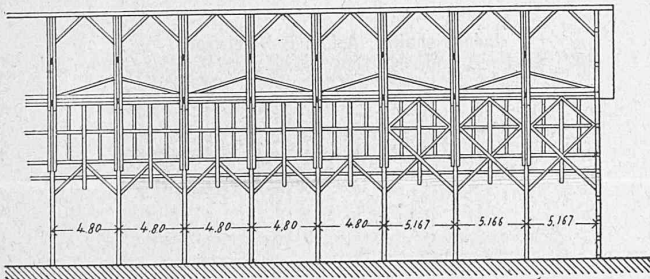
Längenschnitt. Masstab 1:500.
