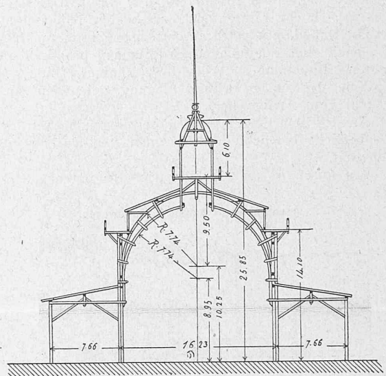
Schnitt. Masstab 1:500.
