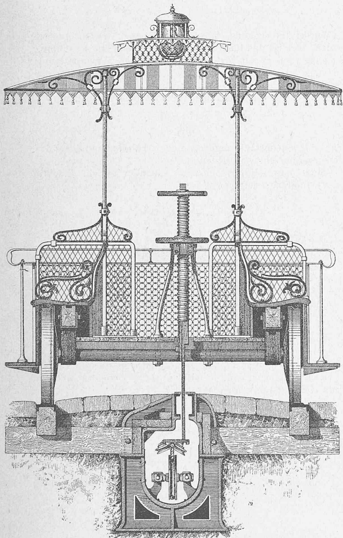
Fig. 3: Querschnitt.
