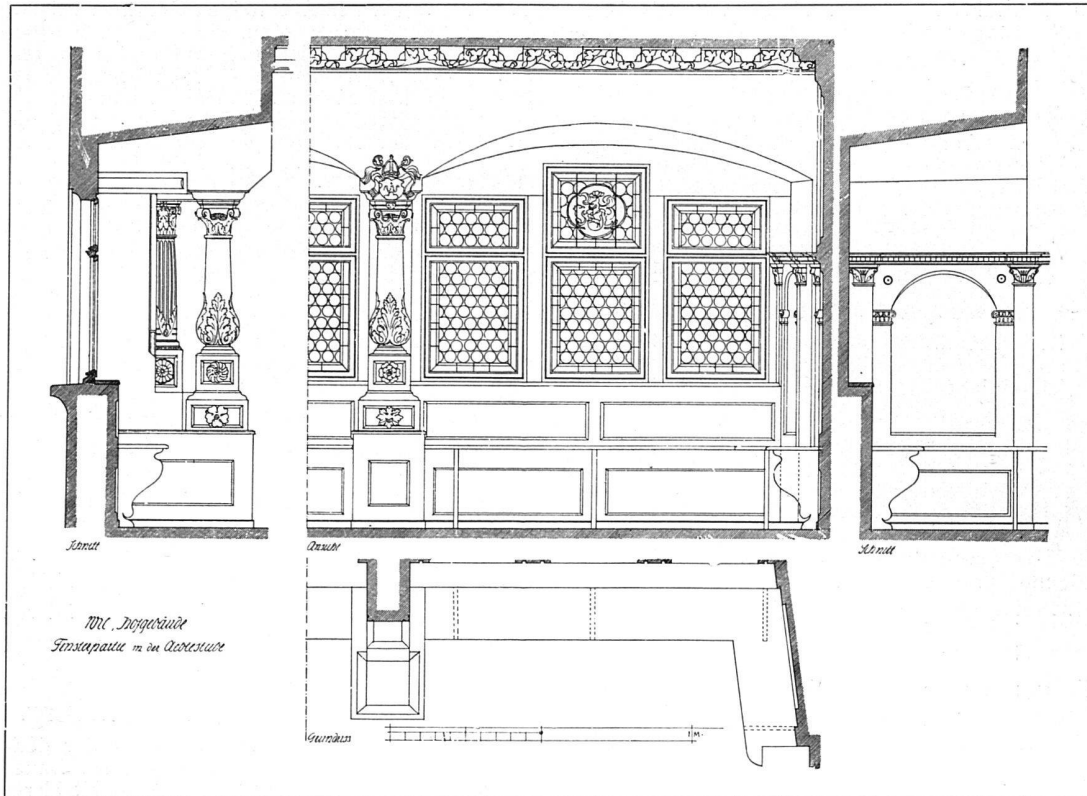
Fensterpartie in der Äbtestube des Hofgebäudes zu Wil (St. Gallen). Massstab 1:50. Aus: Das Bürgerhaus in der Schweiz. Bd. III. St. Gallen (I. Teil) und Appenzell.
