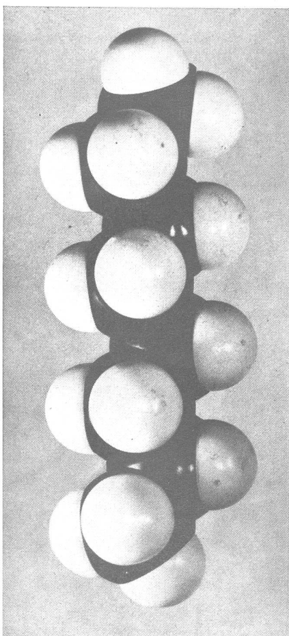
Bild 7: Normal-Octan ( \text{C}_8\text{H}_{18} ) Zickzackform
