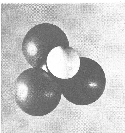
Bild 2: Methan ( \text{CH}_4 )
