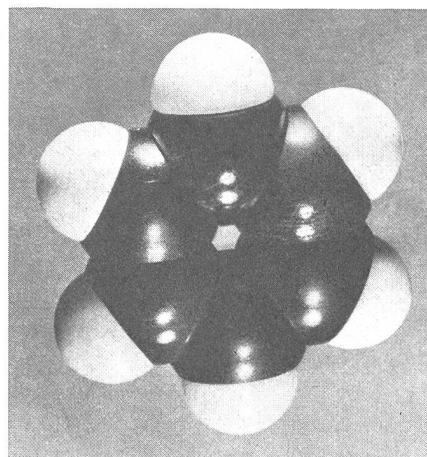
Bild 4: Benzol ( \text{C}_6\text{H}_6 )
