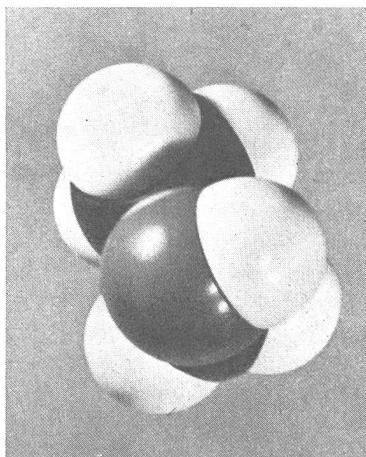
Bild 3: Alkohol ( \text{C}_2\text{H}_5\text{OH} )
