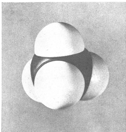
Bild 2: Methan ( \text{CH}_4 )
