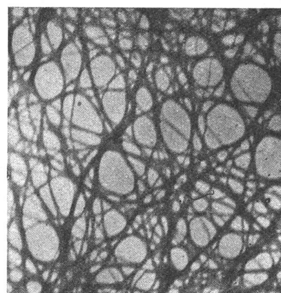
Bild 2 oben: Vanadinpentoxyd-Gel; elektronenoptisch 20 000 : 1.
