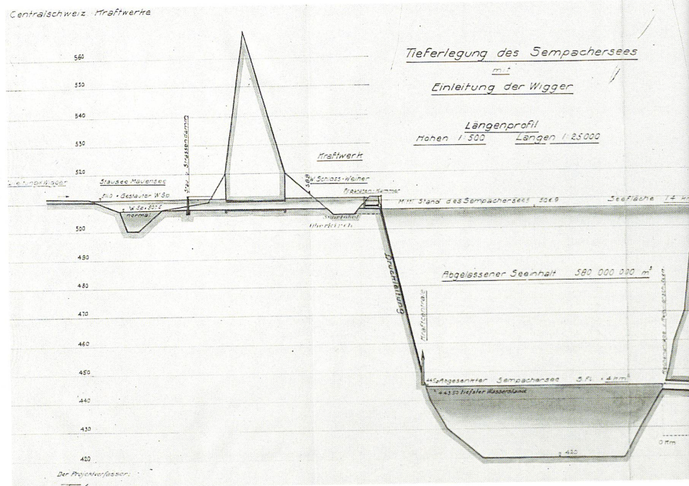
Abb. 4: Längenprofil zum Projekt «Tieferlegung des Sempachersees». Die Staustufe zwischen Mauensee und dem abgesenkten Sempachersee wäre zur Stromgewinnung genutzt und das Wasser
