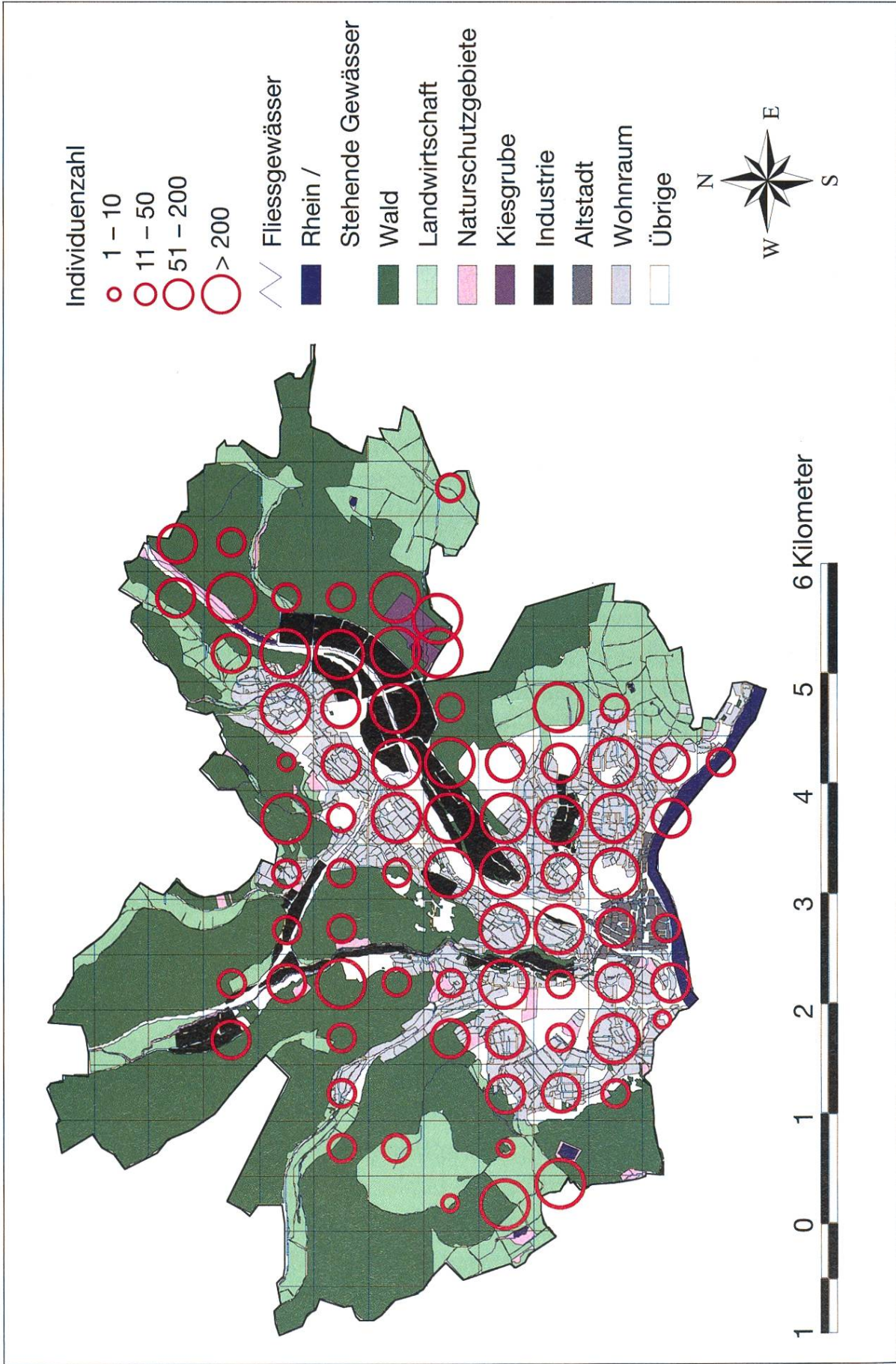
Karte 3: Verbreitung und Individuenzahlen der Kanadischen Golddrute
