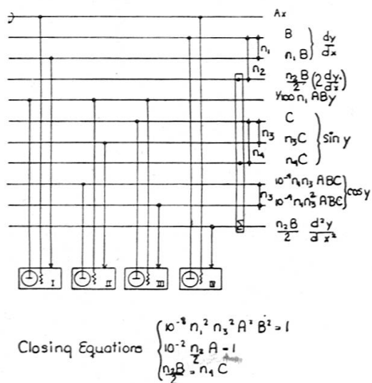
Fig. 13 – Lösung der Differentialgleichung
