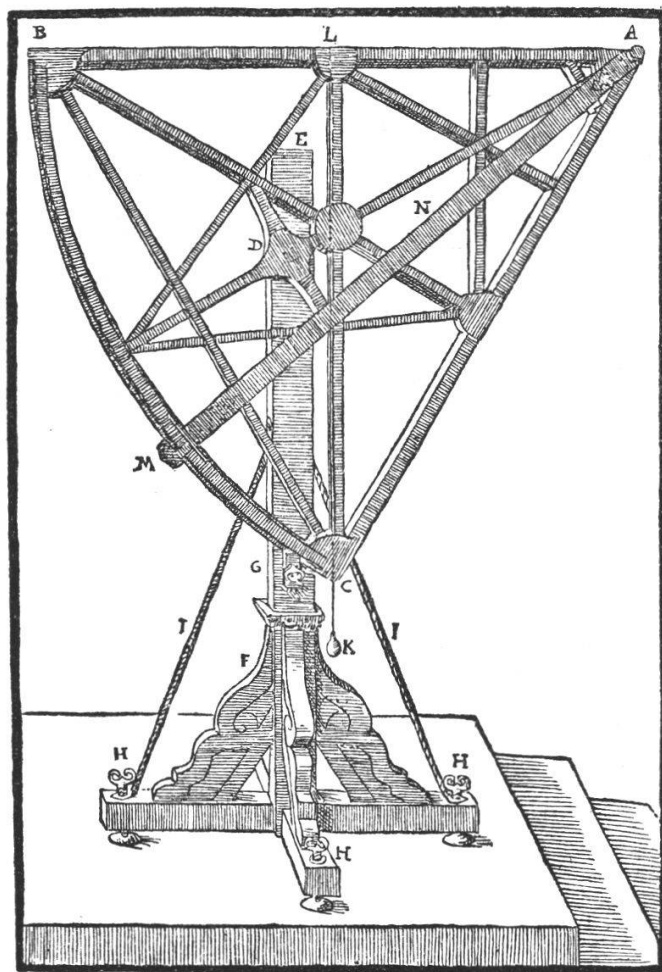
Fig. 3. Astronomischer Sextant.
