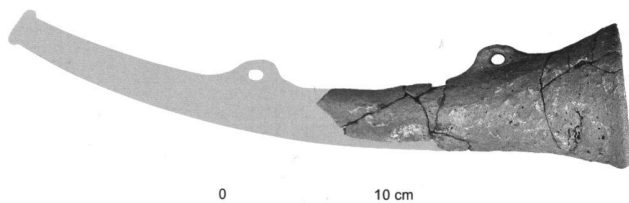
13 : Trompe d'appel découverte sur le flanc du second fossé. Restitution graphique de sa forme complète. – Fragmente einer Signaltrompete aus orange gebranntem Ton (M. 14. Jh.) aus dem zweiten Graben der Burg.
