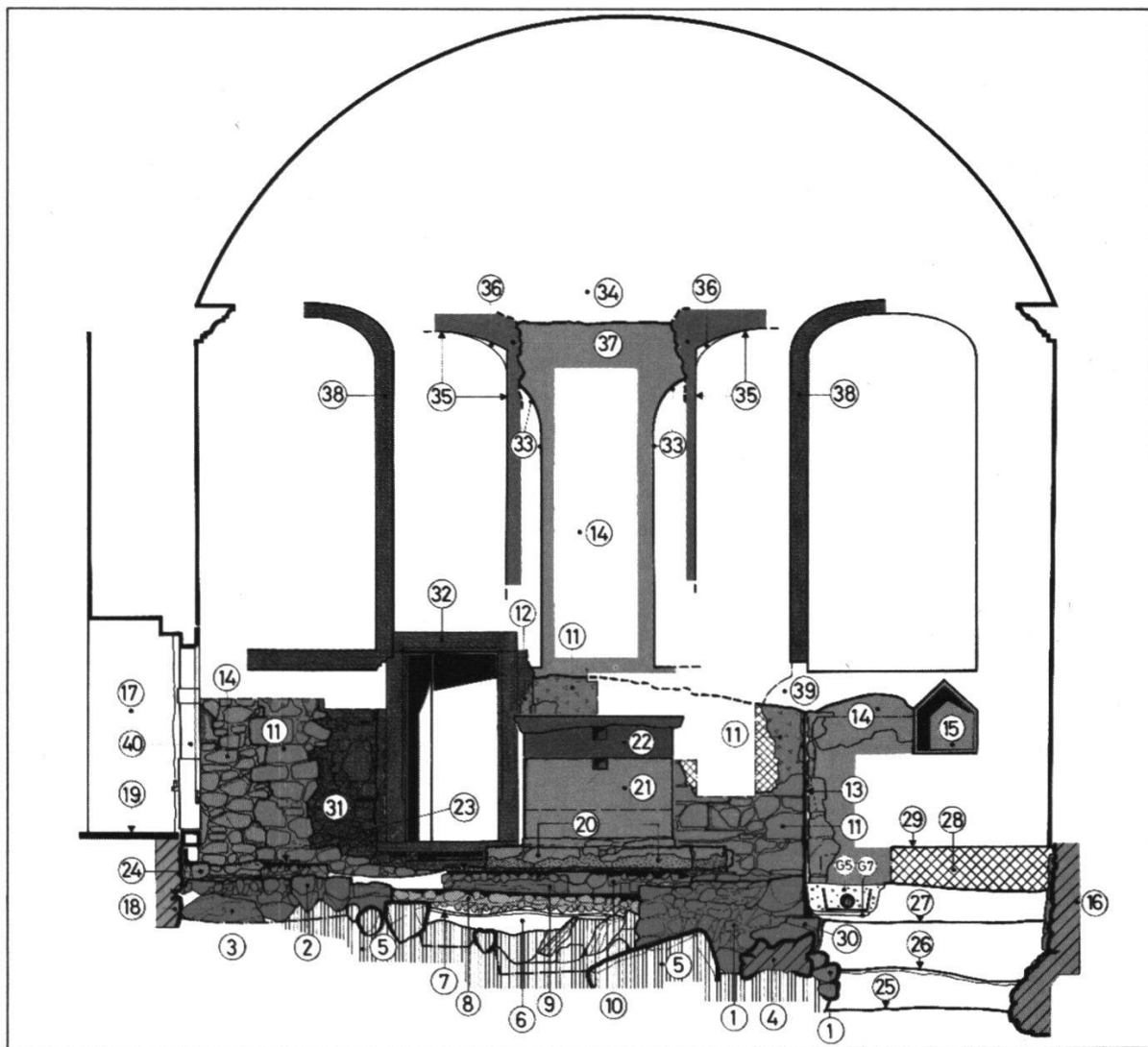
Abbildung 16 Querprofil im Chor mit Ansicht der Chorostwand. Maßstab 1:100. (Farb- legende vgl. Abb. 7) (1) Südliche Chorschulter, Anlage I; (2) nördliche Chorschulter I; (3) nordöstlicher Eckverband des Langhauses I; (4) südliche Langhausmauer I, Schnitt; (5) gewach- sener Boden; (6) Plamierschicht unter dem Apsisboden; (7) Kalkguß unter dem Apsisfuß- boden; (8) Fußboden I auf doppelter Rollierung; (9) Altarfundament I; (10) Fußboden II auf Rollierung; (11) Altarwand II; (12) Reste eines Fensters in Altarwand II; (13) Maueranstoß mit Außenverputz II; (14) Chorostwand III; (15) mit Holz ausgekleidetes Sakraments- häuschen III; (16) Chorsüdmauer III, Schnitt; (17) Südmauer des Glockenturmes IIa; (18) Süd- front des Turmsüdmauer-Fundamentes IIa; (19) Fußbodenniveau im Innern des Turmes; (20) Suppedaneum des Hauptaltars III; (21) Stipes des Hauptaltars III; (22) Aufhöhung des Hauptaltars IIIa; (23) Mörtelstrich des Fußbodens III; (24) Sockelfundament eines Priester- stuhles (?) III; (25) Bauniveau II = unterstes Bauniveau III; (26) zweites Bauniveau III; (27) drittes Bauniveau III, darauf lag eine Schicht aus Abbruchmaterialien der Anlage II; (28) Choraufhöhung von 1928; (29) angetroffenes Fußbodenniveau im Chor, 1928; (30) Stütz- mauer von Chor III (südlicher Teil aus darstellerischen Gründen weggelassen); (31) Mauer der Sakristei von 1796; (32) Türe der Sakristei von 1796; (33) Fensterlaibungen III; (34) Neuauf- mauerung der Giebelwand, 17. Jh.; (35) Fensterlaibungen der Barockisierung, 1718/20; (36) aufgetragene Gipsglätte, 1777; (37) Ausbruch bei der Anlage der barocken Fenster, 1718/20; (38) Stuckrahmen der aktuellen Fenster, mit der Errichtung der Sakristei 1796 angelegt; (39) Ausbruch bei der Anlage der aktuellen Fenster, 1796; (40) östliches Gewände des auf das Jahr 1585 datierten Turmportals, 1827/28 beim Abbruch der alten Sakristei vor die Südfassa- de des Turmes gesetzt.
