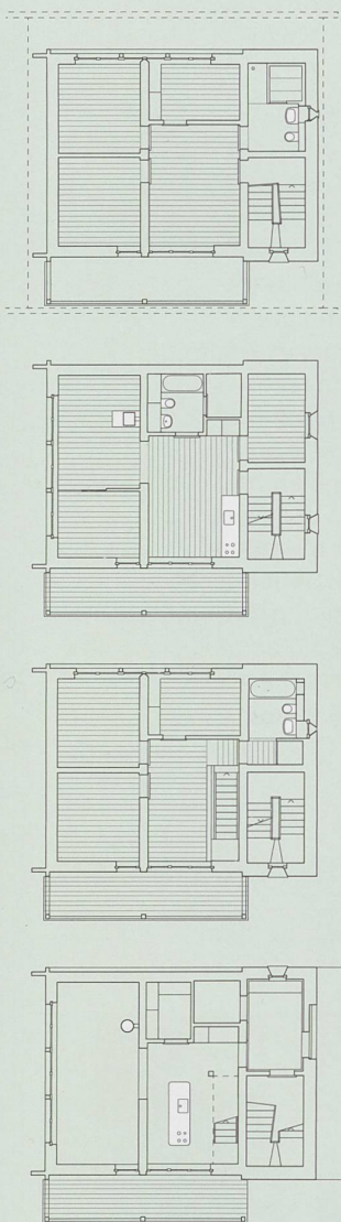
Fig. 1 Coupe et plans des étages du chalet Jaccaud-Zein. © bureau JSAA, 2015
