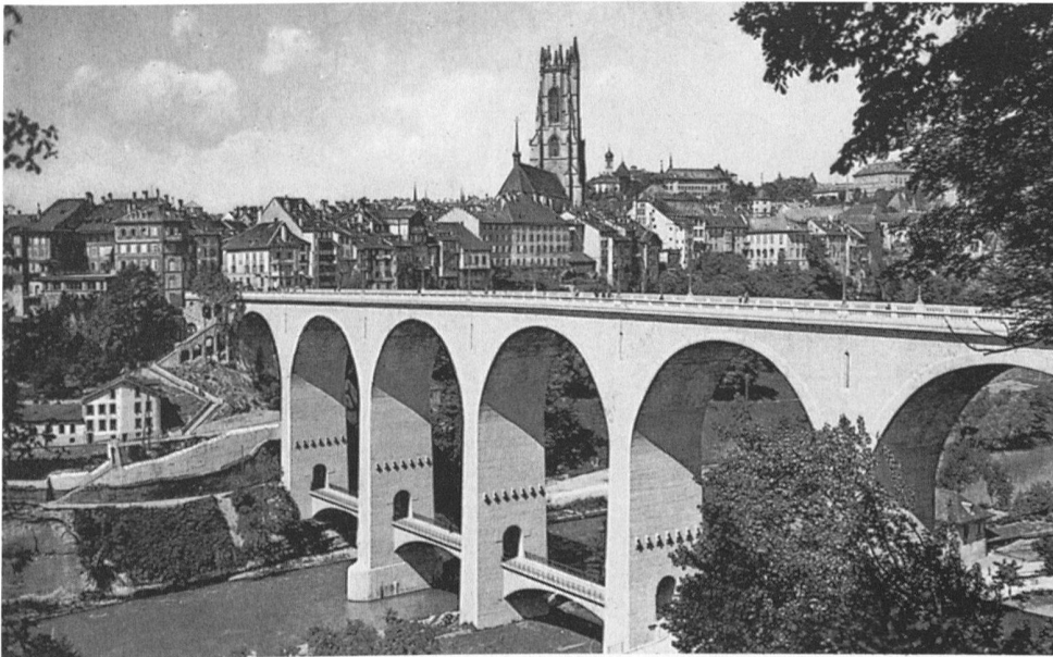
5 Die 1923–1924 erbaute Zähringerbrücke ersetzte den «Grand Pont», der im April 1924 abgebrochen wurde. Dafür erhielt im unteren Geschoss das Au-Quartier einen weiteren Saaneübergang.
