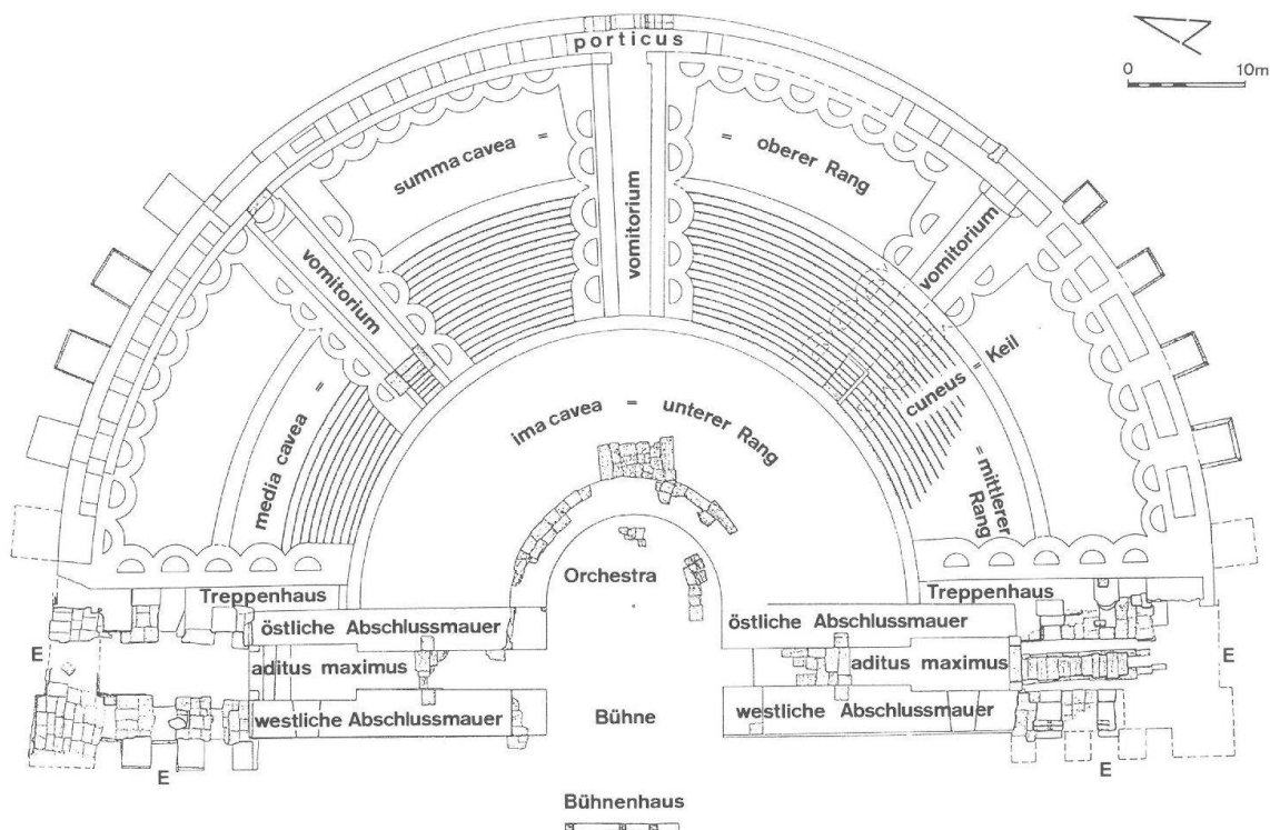
Abb. 1 Augst BL, Theater. Grundriss des dritten Theaters mit Bezeichnungen wichtiger Bauteile. M. 1:700.
