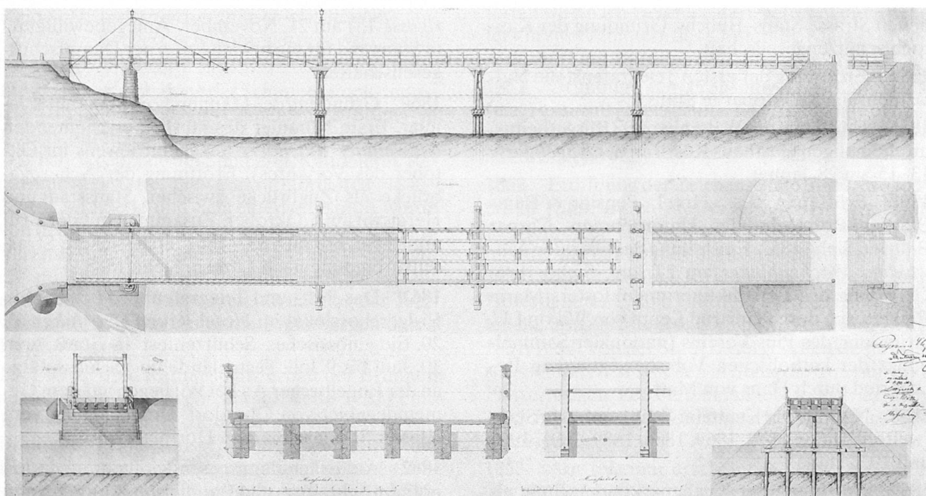
Abb. 4 Plan der ersten Achereggbrücke von 1860. Die Zugbrücke ermöglicht die direkte Verbindung zwischen Stansstad und Hergiswil.
