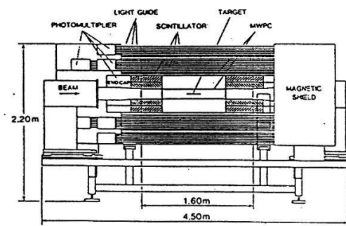
Fig. 1 LADS Längsschnitt
