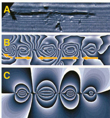
A. Image holographique réalisée à l'aide d'un microscope électronique à transmission. Au centre, on voit un nanofil (longueur: 6 millièmes de millimètre). Les franges qui l'entourent résultent d'interférences produites par deux faisceaux d'électrons.
