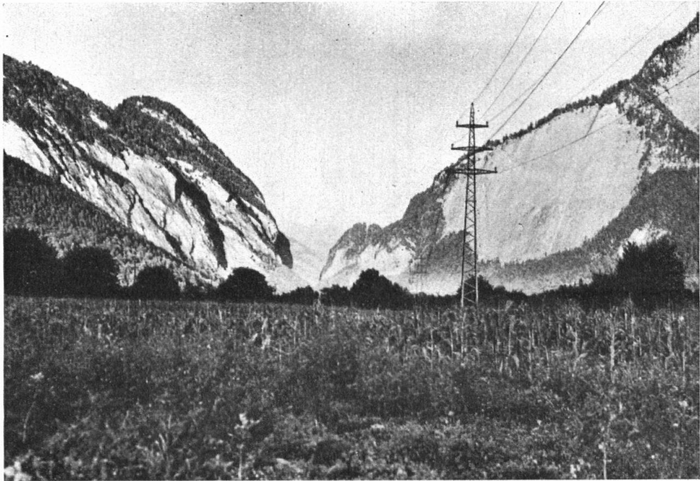
Abb. 12. Eleganter Eisengittermast der B. K. am Ausgange der Klus. Die dauerhaft feuerverzinkten Oberteile sind in drei Jahren bereits stärker abgedunkelt als die mit Oelfarbe gestrichenen Unterteile der Masten und deshalb oft weit weniger sichtbar als letztere. — Fig. 12. Pylône élégant de la B. K. à la sortie des gorges de la Clus. Les parties supérieures en fer galvanisé prennent au bout de 3 ans une couleur plus foncée que les parties inférieures peintes à l'huile, aussi sont-elles moins apparentes que celles-ci.
