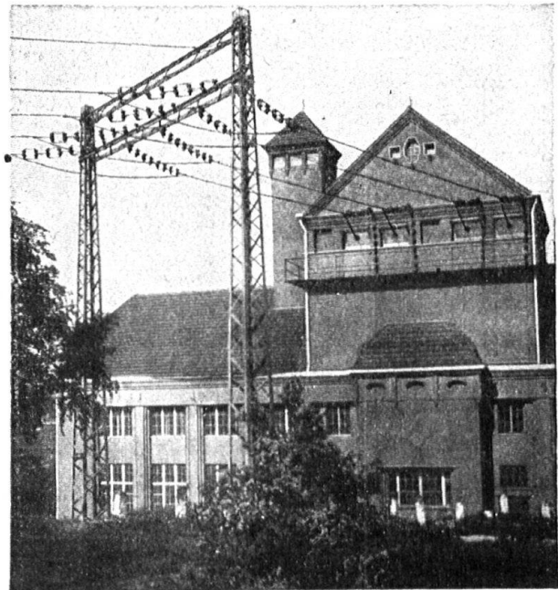
Abb. 3. Eintritt einer Oberspannungsleitung für 100,000 Volt in eine Transformatorenstation. Das riesenhafte Joch zerstört durch seine scharfen Überschneidungen die Harmonie der guten Architektur. Cliché der Elektrotechnischen Zeitschrift, Berlin 1919. — Fig. 3. Comment une conduite électrique à haute tension est reliée à une station transformatrice. Ce pylône colossal aux formes disgracieuses forme un contraste désagréable avec les lignes harmonieuses du transformateur. Cliché de l'« Elektrotechnische Zeitschrift », 1919.
