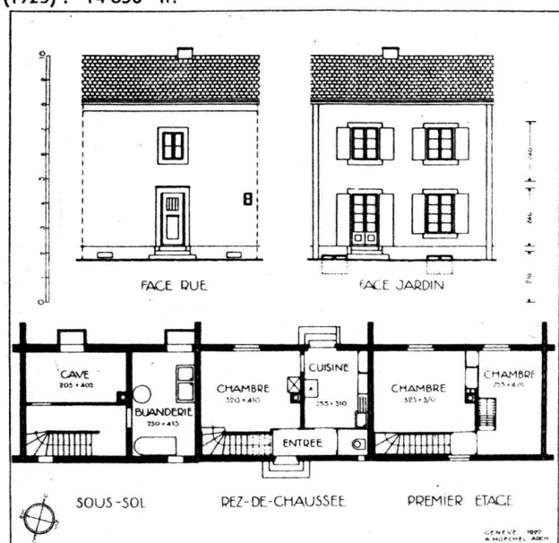
Plan et façade d'une maison des deux groupes construits en 1922-1923. Habitations de 3 chambres et cuisine, baaignoire dans la buanderie. Voir photo du haut. Surface : 33 m 2 . Volume : 303 m 3 . Prix : 12 380 fr.
