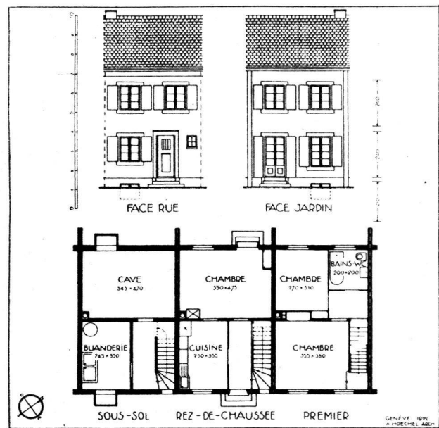
Plan et façade d'une maison des huit groupes de 1920 à 1923. Habitations de trois chambres, cuisine et salle de bains. Service d'eau chaude. Chaque groupe comprend quatre maisons semblables. Un neuvième groupe en comprend six. Surface : 38 m 2 . Volume : 359 m 3 . Prix (1921) : 18 910 fr. (1923) : 14 850 fr.
