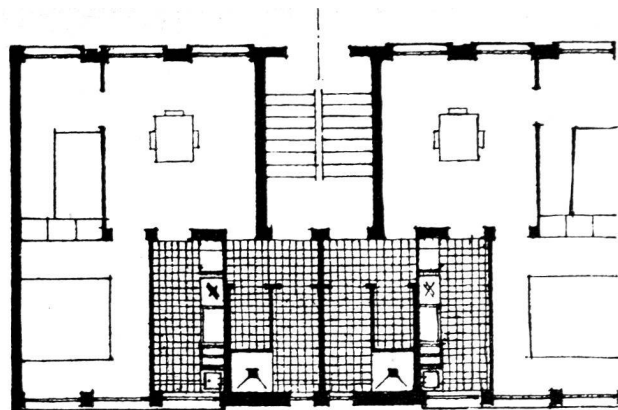
Plan du rez-de-chaussée et des étages du groupe B de la Cité-Vieusseux.
