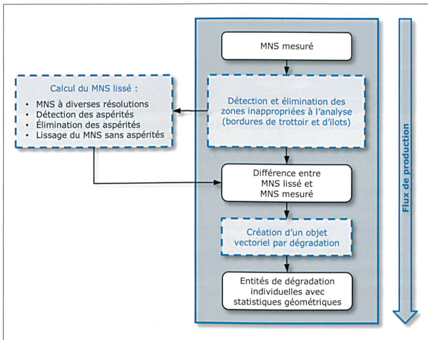
Fig. 4: Principe de détection des dégradations et des déformations. Abb. 4: Prinzip der Ortung der Abnutzungen und Verformungen. Fig. 4: Principio di detezione del degrado e della deformazione.
