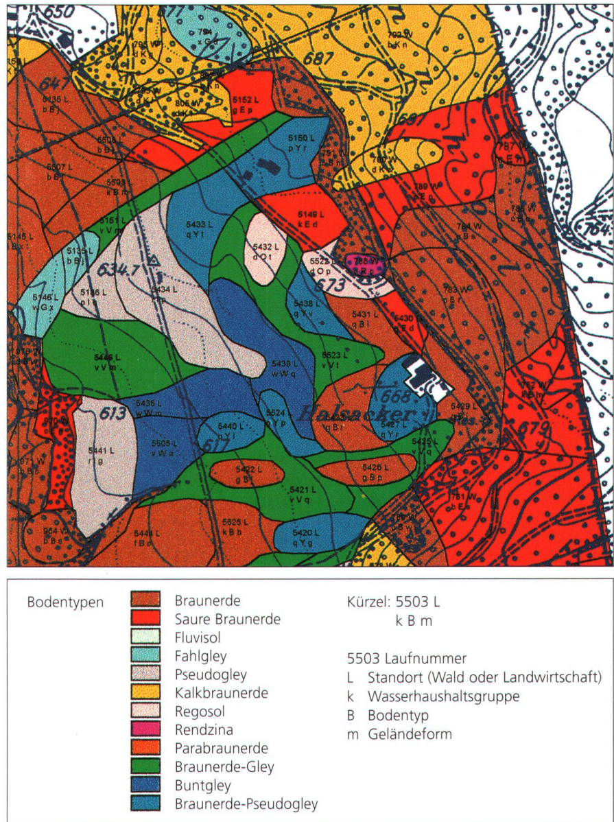
Abb. 3: Informationssystem Boden. Ausschnitt aus der Ebene Bodentypen. (Reproduziert mit Bewilligung des Kantonalen Vermessungsamtes Solothurn vom 7.4.97.)
